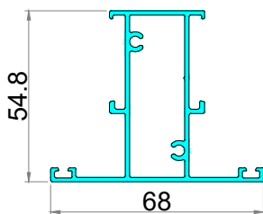
Đố chữ T cho khung cố định
