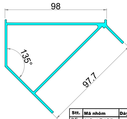
Ghép khung bao hệ 55
