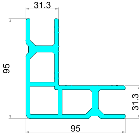
Liên kết góc khung bao, cánh cửa đi
