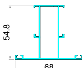
Đố chữ T cho khung cánh
