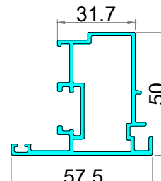
Đố động dùng chung
